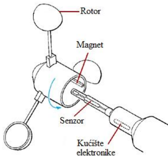
Slika 8. Shematski prikaz anemometra (izvor: Peet Bros. 2018. Anemometer. Dostupno sa: http://www.peetbros.com/shop/custom.aspx?recid=17 , pristupljeno: svibanj 2018. godine)
