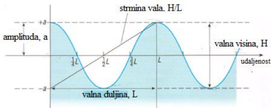
Slika 1. Vertikalni profil dva uzastopna idealizirana morska vala koji prikazuje dimenzije valova i njihov sinusoidalni oblik (izvor: prema Wright i sur., 1999).
