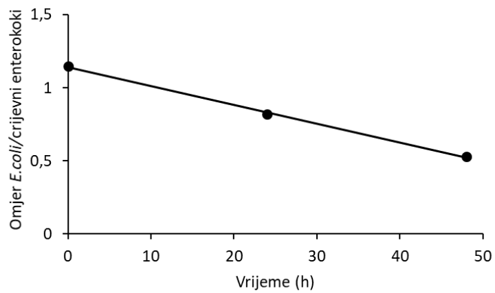
Slika 13. Promjena omjera E.coli /crijevni enterokoki tijekom prvog in situ eksperimenta u odsutnosti Sunčevog svjetla
