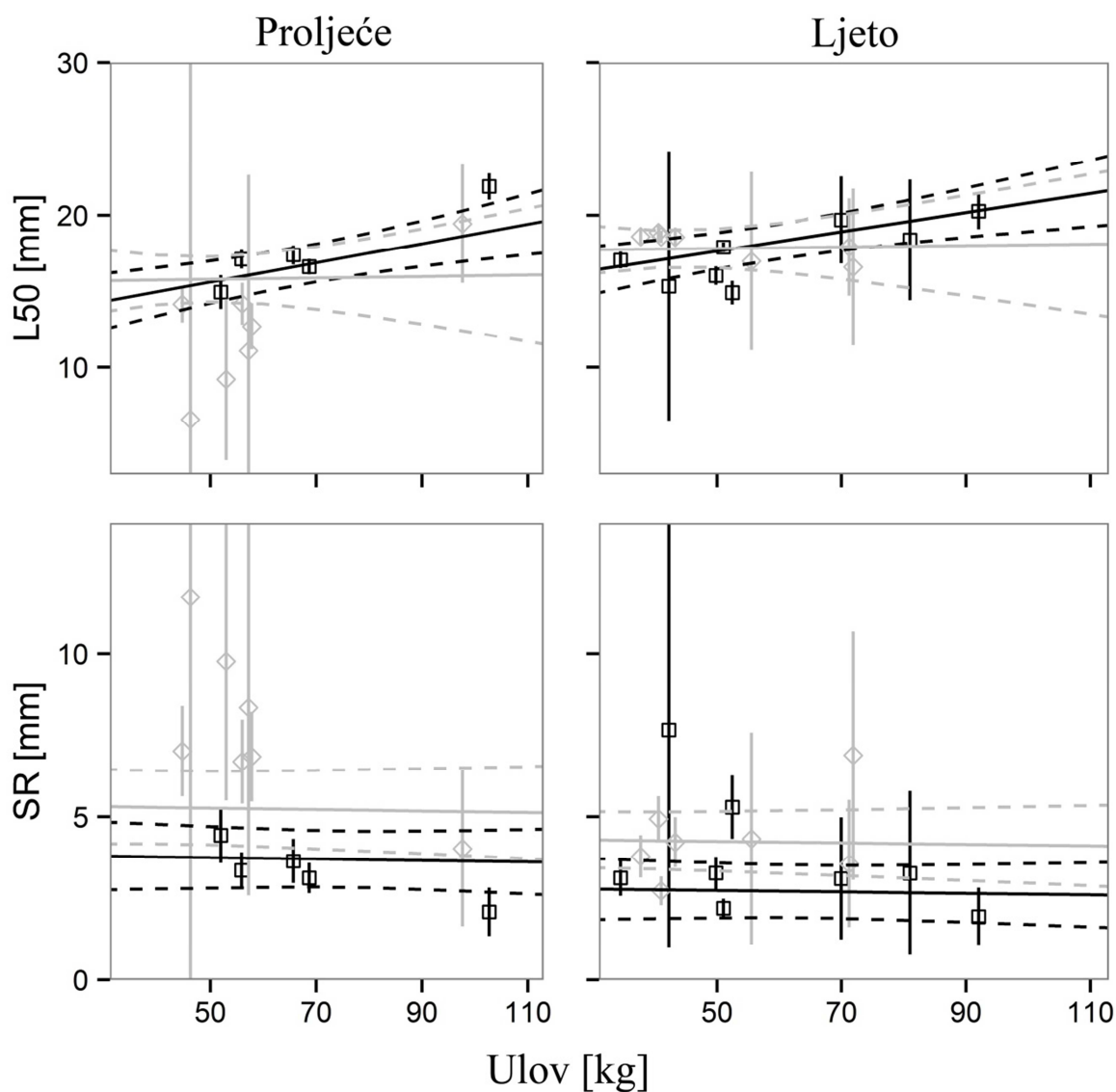
Slika 4.12. Predikcija selekcijskih parametara L50 i SR za vrstu P. longirostris u ovisnosti o količini ulova u vreći mreže. Isprekidane sive linije predstavljaju 95-postotne intervale povjerenja predikcijske krivulje KV40 vreće (puna siva linija). Isprekidane crne linije predstavljaju 95-postotne intervale povjerenja predikcijske krivulje RO50 vreće (puna crna linija). Crni i sivi kvadratni simboli predstavljaju srednje vrijednosti selekcijskih parametara individualnih potega KV40 i RO50 vreće, a vertikalne crne i sive linije predstavljaju njihove 95-postotne intervale povjerenja.
