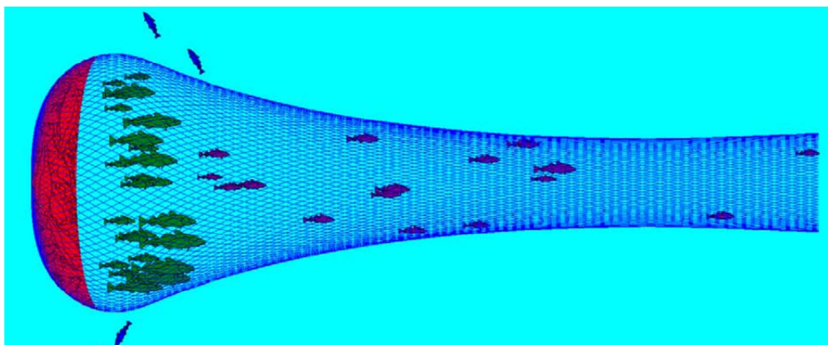
Slika 2.1. Različita otvorenost mrežnih oka pri povlačenju vreće izrađene od kvadratnog oka (Izvor: Herrmann, 2005).
