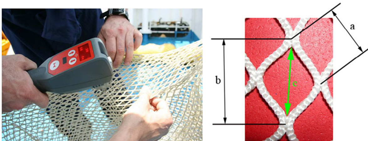
Slika 3.3. OMEGA mjerač oka mrežnog tega upotrebljavan u istraživanjima (lijevo). Različiti načini označavanja dimenzija mrežnog oka (desno): a – dužina jedne stranice oka; b – veličina oka; c – otvor oka.
