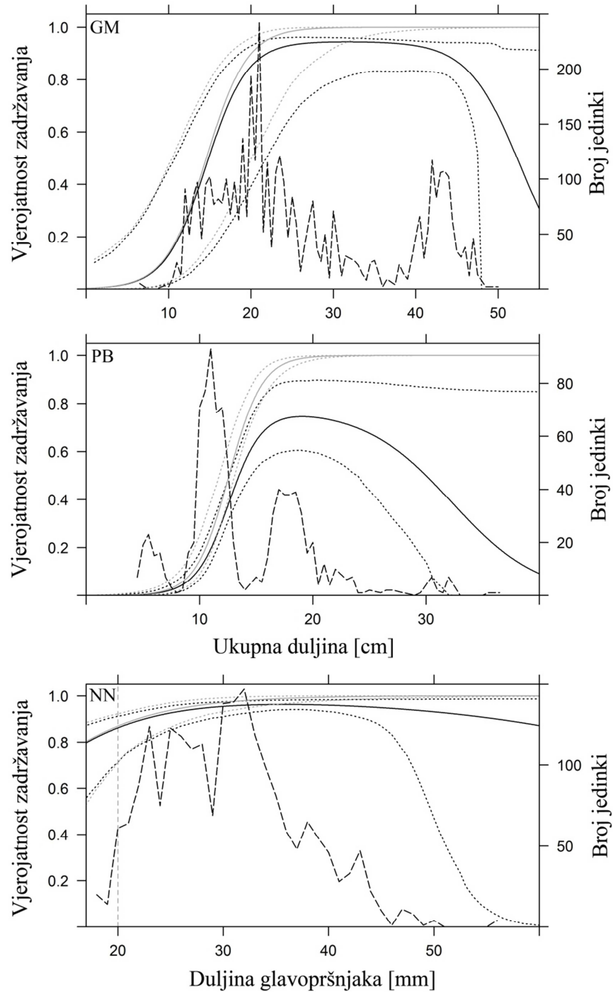
Slika 4.22. Usporedba selektivnosti eksperimentalnog koćarskog sustava sa i bez selektivne rešetke (samo vreća). Puna crna linija predstavlja krivulju selekcijskog sustava s rešetkom, a točkaste crne linije njihove 95-postotne intervale povjerenja. Siva puna linija predstavlja krivulju selekcijskog sustava bez selektivne rešetke, a točkaste sive linije njihove 95-postotne intervale povjerenja. Iscrtkana crna linija predstavlja strukturu populacije koja je naišla na alat tijekom ribolova. Vertikalna iscrtkana siva linija predstavlja minimalnu lovnu duljinu vrste. GM: G. melastomus , NN: N. norvegicus and PB: P. blennoides .
