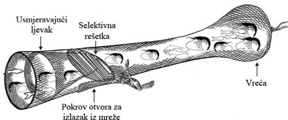
Slika 2.10. TED - Selektivna rešetka pomoću koje se oslobađaju morske kornjače iz ulova (Izvor: FAO, 2009).
