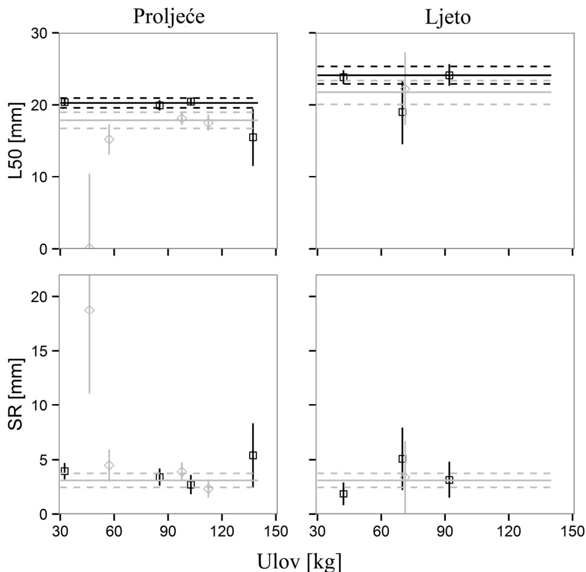
Slika 4.8. Predikcija selekcijskih parametara L50 i SR za vrstu N. norvegicus u ovisnosti o količini ulova u vreći mreže. Isprekidane sive linije predstavljaju 95-postotne intervale povjerenja predikcijske krivulje KV40 vreće (puna siva linija). Isprekidane crne linije predstavljaju 95-postotne intervale povjerenja predikcijske krivulje RO50 vreće (puna crna linija). Crni i sivi kvadratni simboli predstavljaju srednje vrijednosti selekcijskih parametara individualnih potega KV40 i RO50 vreće, a vertikalne crne i sive linije predstavljaju njihove 95-postotne intervale povjerenja.
