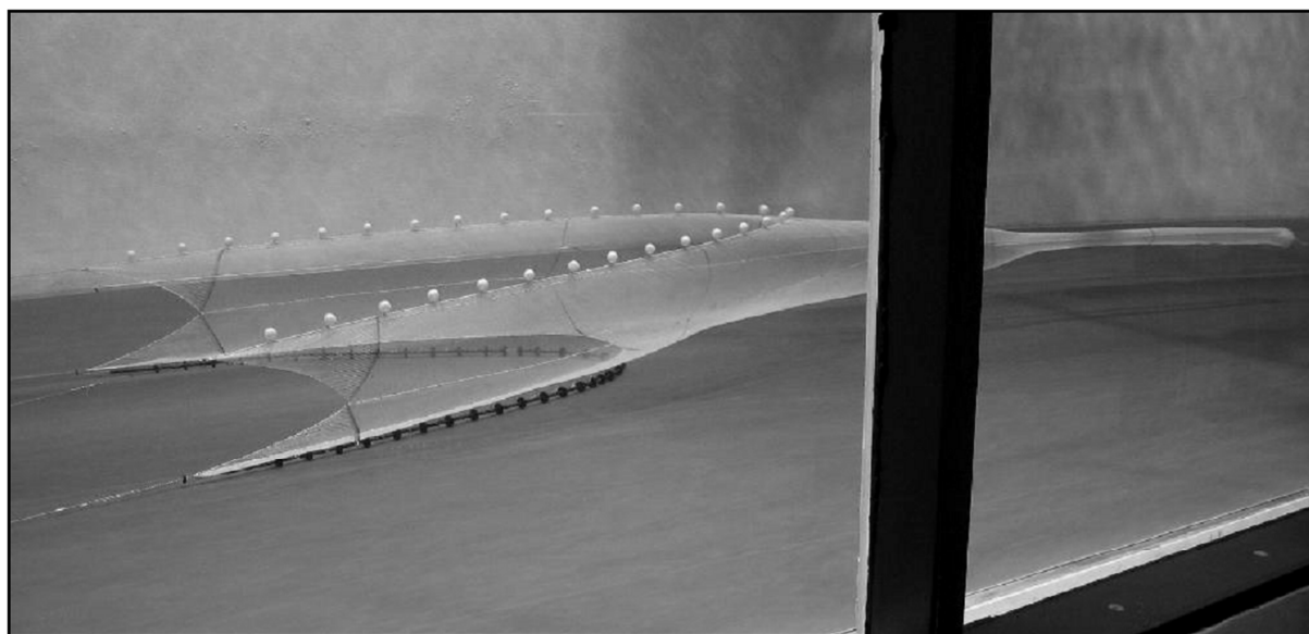
Slika 2.13. Model pridnene povlačne mreže koće kojoj je u potpunosti uklonjeno nebo i prednji dio grla (Izvor: He & Goethel, 2007).
