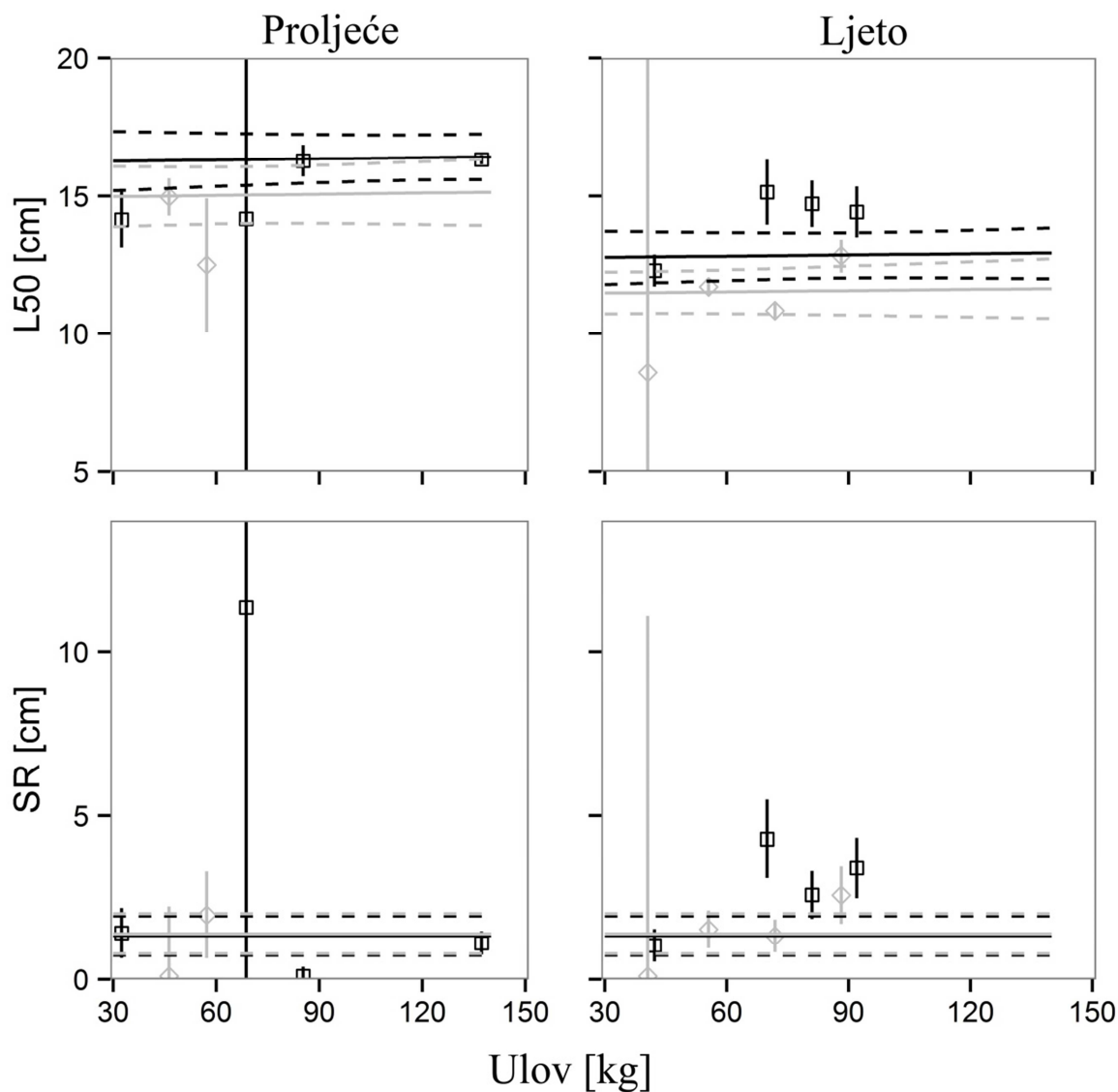
Slika 4.10. Predikcija selekcijskih parametara L50 i SR za vrstu P. blennoides u ovisnosti o količini ulova u vreći mreže. Isprekidane sive linije predstavljaju 95-postotne intervale povjerenja predikcijske krivulje KV40 vreće (puna siva linija). Isprekidane crne linije predstavljaju 95-postotne intervale povjerenja predikcijske krivulje RO50 vreće (puna crna linija). Crni i sivi kvadratni simboli predstavljaju srednje vrijednosti selekcijskih parametara individualnih potega KV40 i RO50 vreće, a vertikalne crne i sive linije predstavljaju njihove 95-postotne intervale povjerenja.
