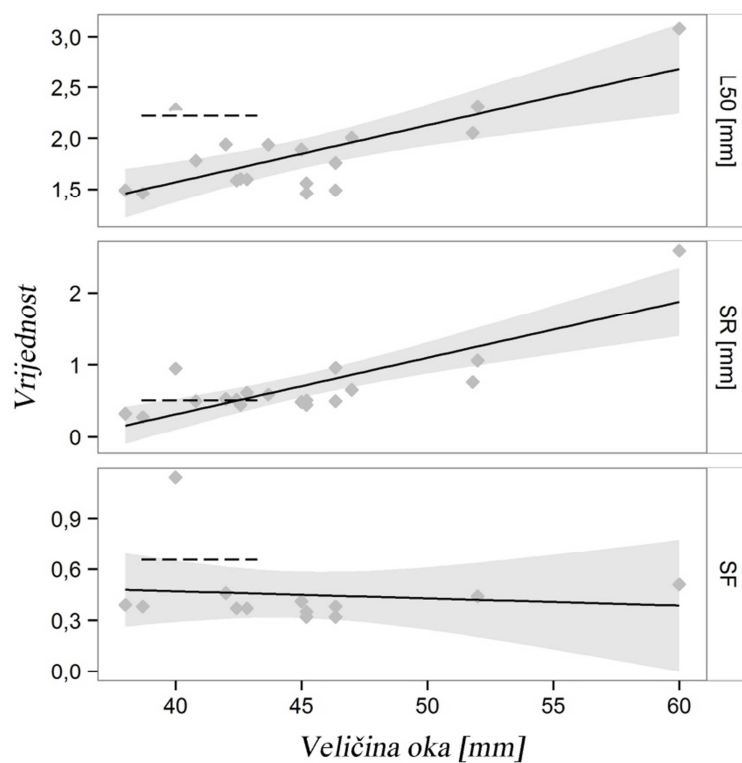
Slika 4.60. Odnos između selekcijskih parametara (L50, SR, SF) i veličine oka za vrstu N. norvegicus . Puna linija predstavlja vreću izrađenu od romboidnog, dok isprekidana linija predstavlja vreću izrađenu od kvadratnog mrežnog oka. Za kvadratno oko prikazana je samo srednja vrijednost parametara zbog malog broja provedenih studija.
