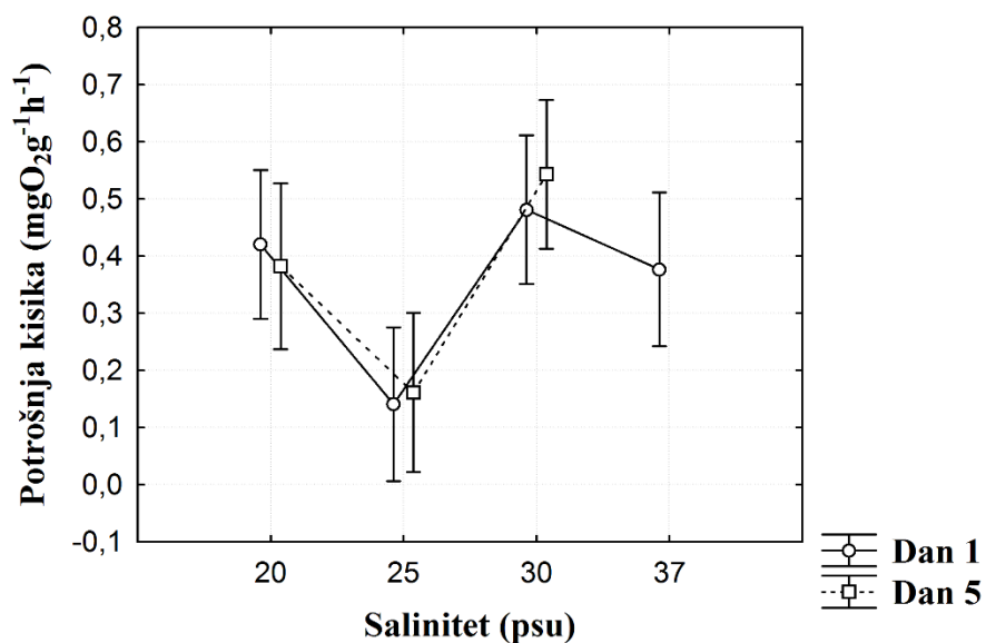
Slika 4.1.1.1.1. Odnos potrošnje kisika i saliniteta morske vode kod kunjke tijekom prvog i petog dana izlaganja.
