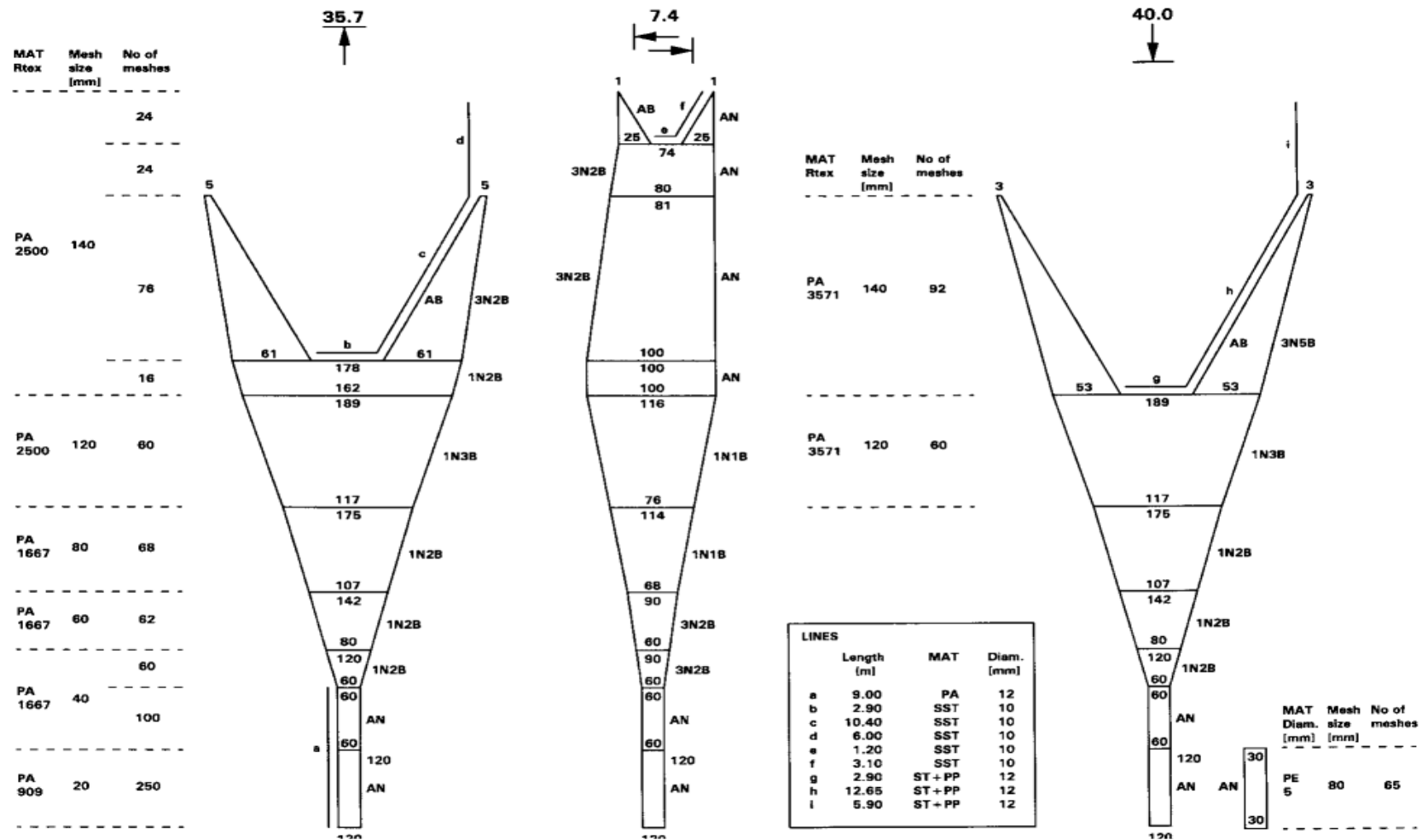
Slika 2.2.2. Shematski prikaz pridnene povlačne mreže koće tipa GOC 73 korištene tijekom istraživanja u okviru MEDITS projekta (izvor: Bertrand i sur., 2002).
