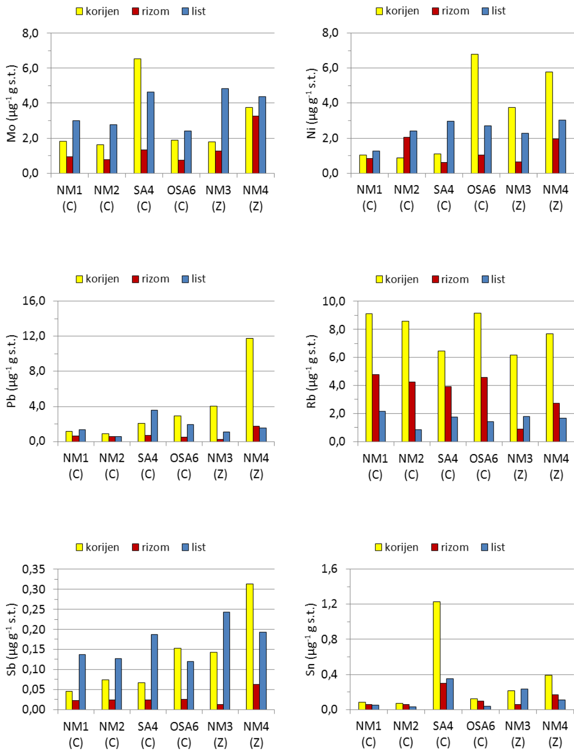
Slika 5.9.4. Maseni udjeli Mo, Ni, Pb, Rb, Sb i Sn u korijenju, rizomima i lišću vrsta C. nodosa (postaje s oznakom C) i Z. noltei (postaje s oznakom Z).
