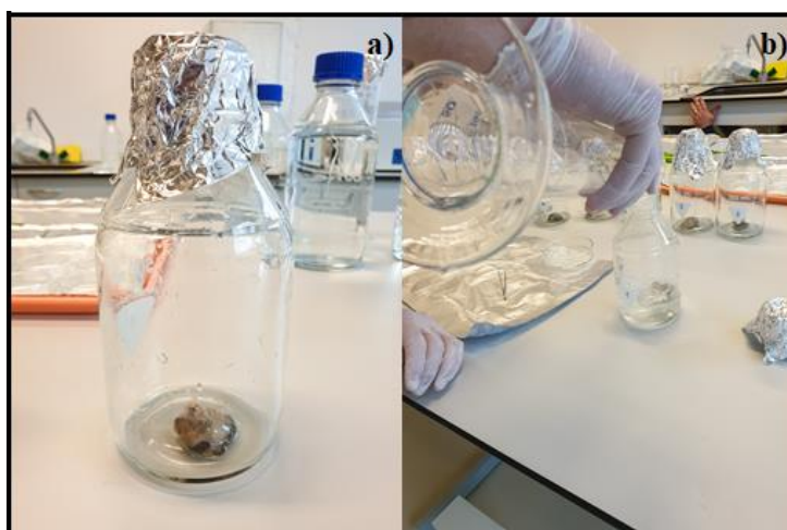
Slika 15. a) Stavljanje čitavog tkiva vrste Ostrea edulis u konusnu tikvicu b) Dodavanje H_2O_2 u konusnu tikvicu s tkivom (slika: E. Vranjić).
