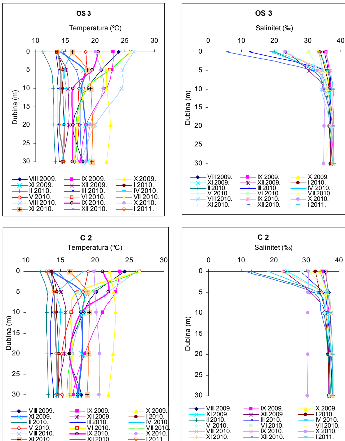
Slika 5.1.2. Raspodjela temperature ( ^{\circ}\text{C} ) i saliniteta ( \text{‰} ) na području Tivatskog zaljeva
