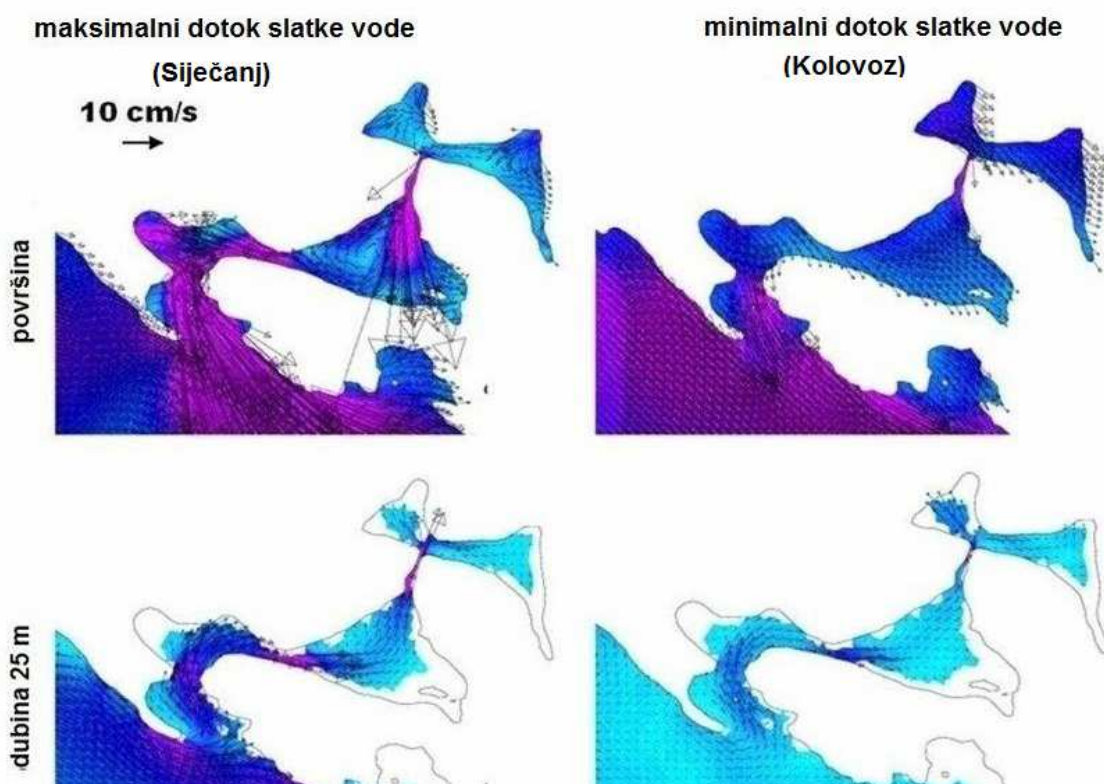
Slika 4.1.3. Generalni model morskih struja: površina (gornja slika) i dubina 25 m (donja slika) u Bokotorskom zaljevu za različitu dinamiku dotoka slatke vode (siječanj i kolovoz) (izvor: Bellafiore i sur. 2011)
