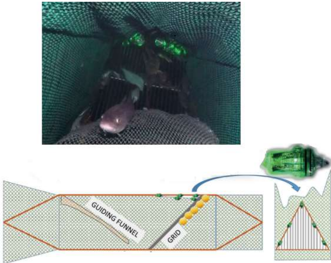
Slika 7. LED svjetla postavljena oko otvora iznad Nordmöre rešetke (Izvor: Larsen i sur., 2017).
