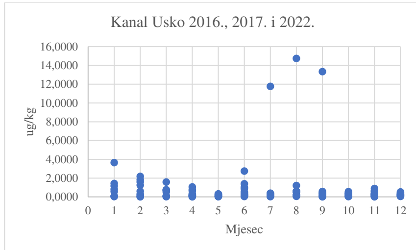
Slika 23. Raspodjela vrijednosti spiorolida tijekom tri godine u 12 mjeseci na postaji Kanal Usko.
