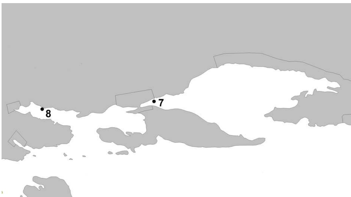
Slika 7. Područje istraživanja po kontrolnim točkama u Kaštelanskom i Marinskom zaljevu.
