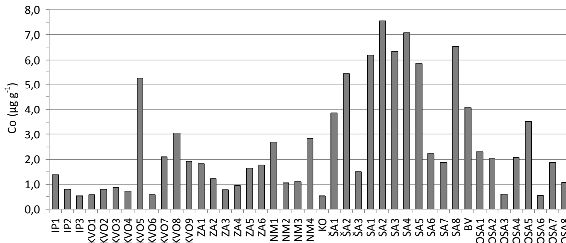
Slika 5.5.9. Maseni udjeli kobalta ( \mu\text{g g}^{-1} ) u površinskim sedimentima istraživanog područja.
